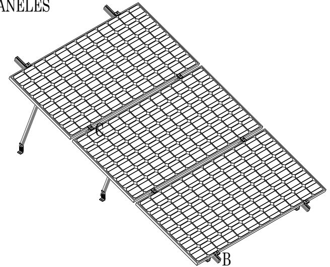
VISTA ISOMÉTRICA
