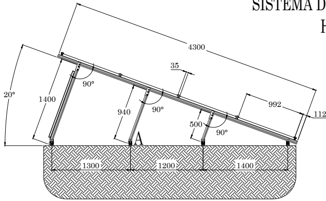
VISTA LATERAL
