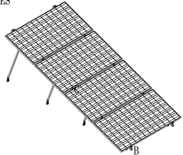
VISTA ISOMÉTRICA
