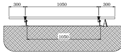
VISTA LATERAL
