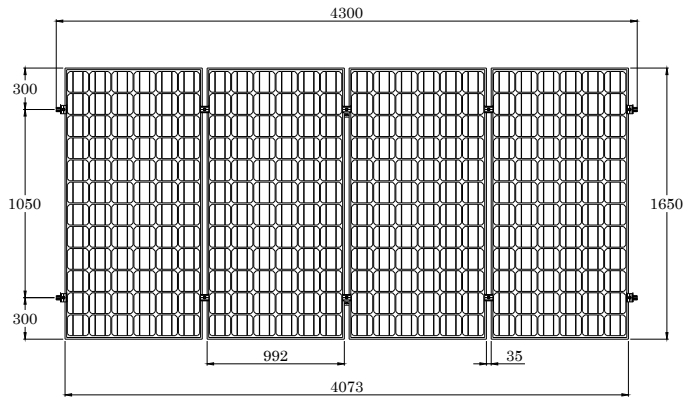
VISTA PLANTA
